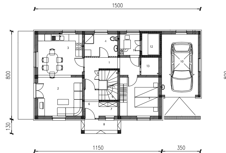
PRITLIČJE 1 : 200
