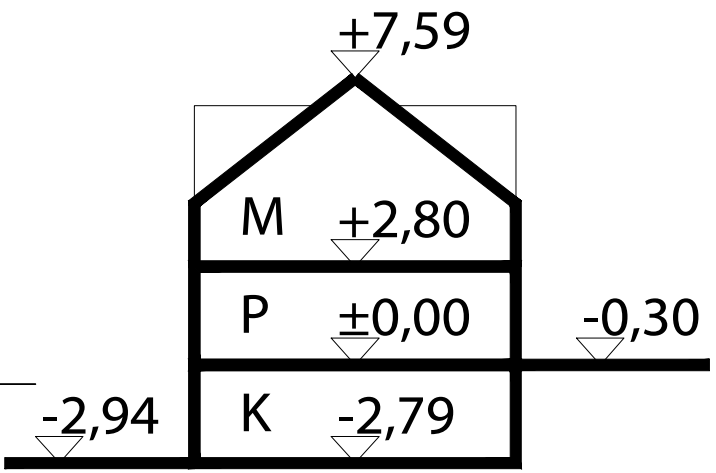
PREČNI PREREZ
