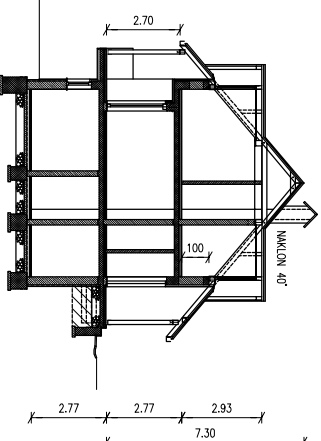
PREČNI PREREZ
