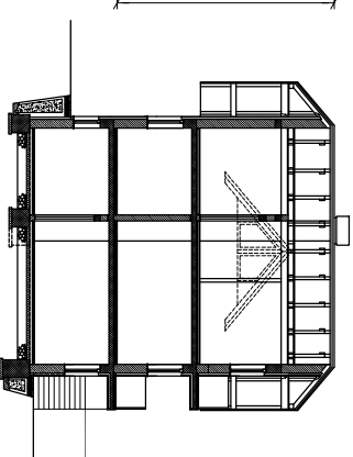
VZDOLŽNI PREREZ
