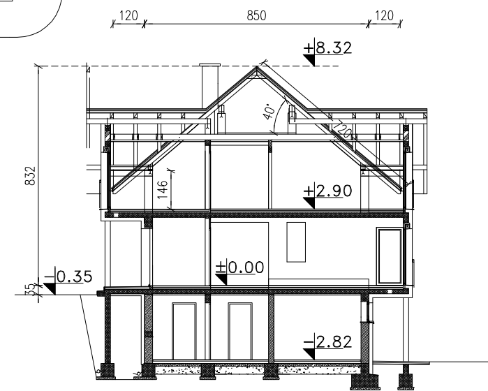
PREREZ M1:200
