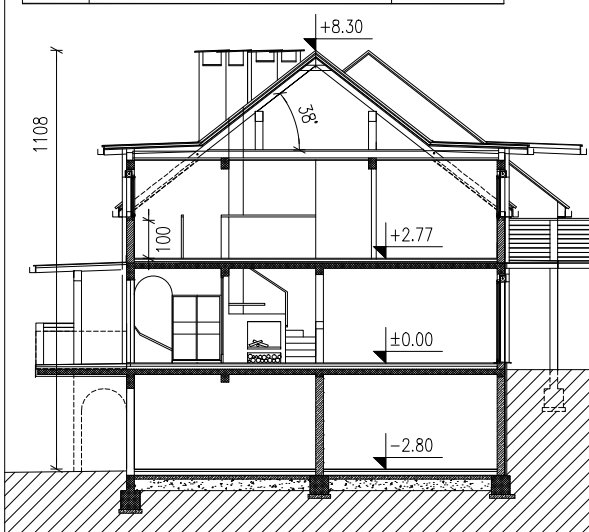
PREREZ 1:200
