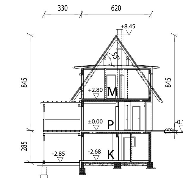
PREČNI PREREZ M=1:200
